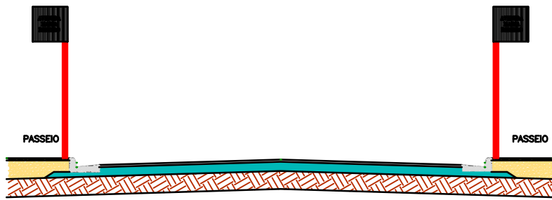
DETALHE DAS ESTRUTURA DO PAVIMENTO
