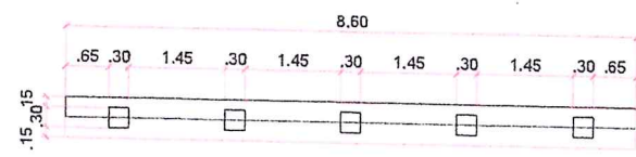
PLANTA - BLOCO CONCRETO ARMADO
