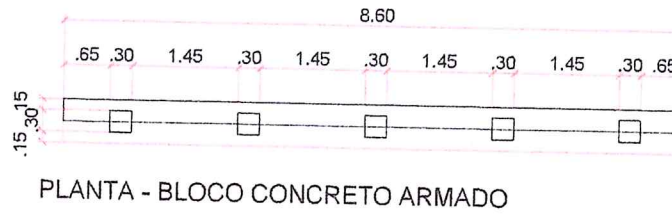
PLANTA BLOCO S/ESC.
