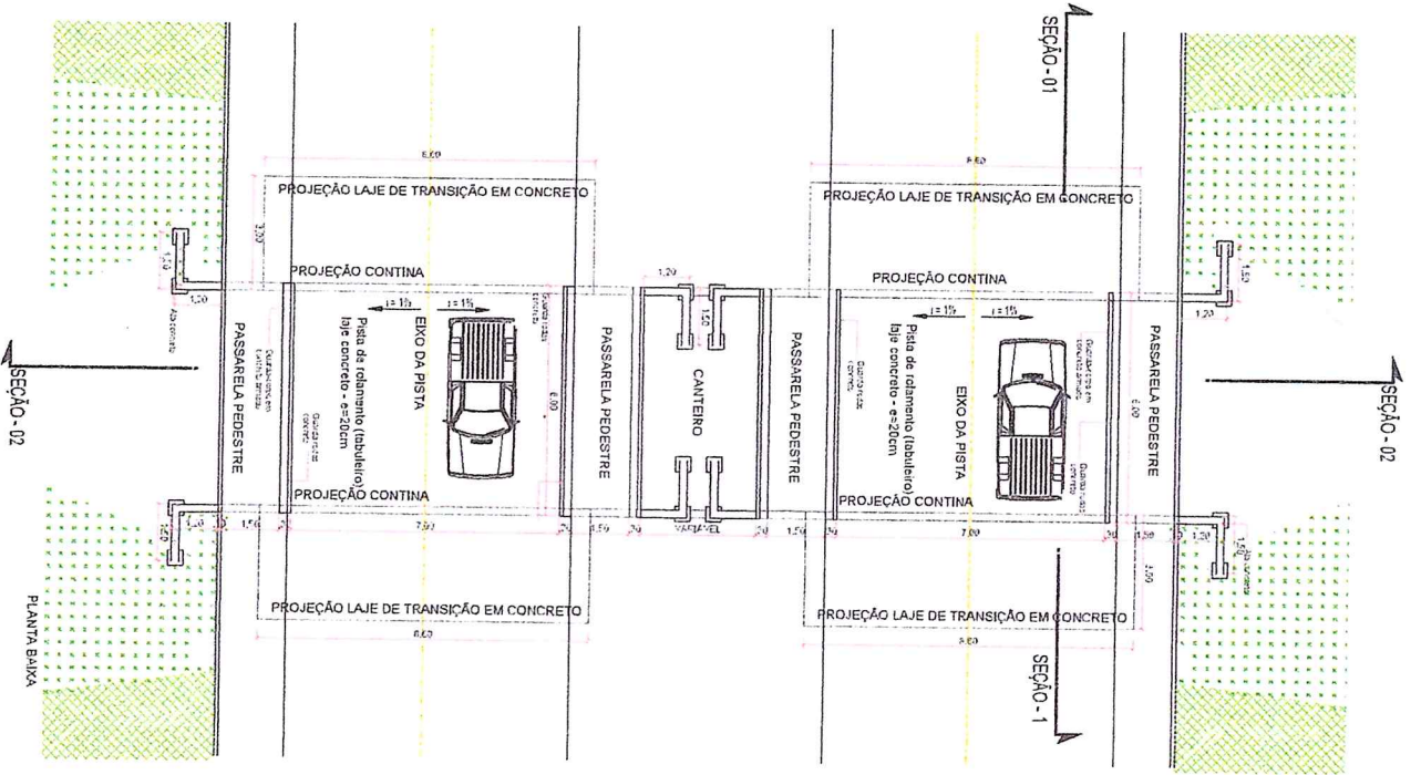
PLANTA BAIXA AV BRASIL ESC. 1/75
