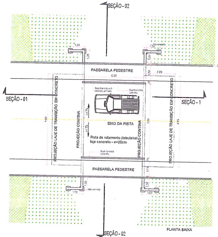
PLANTA BAIXA RUA CURITIBA ESC. 1/75
