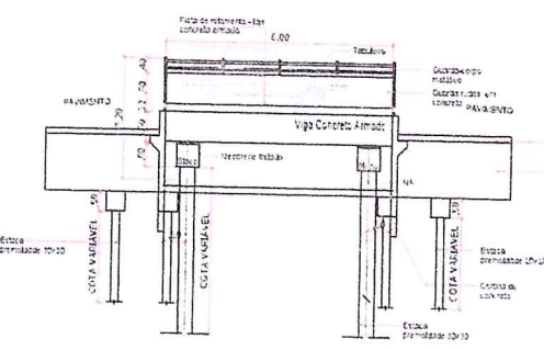
SEÇÃO 01 ESC. 1/100
