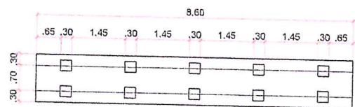
PLANTA - BLOCO CONCRETO ARMADO
