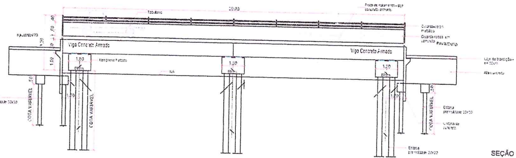
SEÇÃO 01 ESC. 1/100
