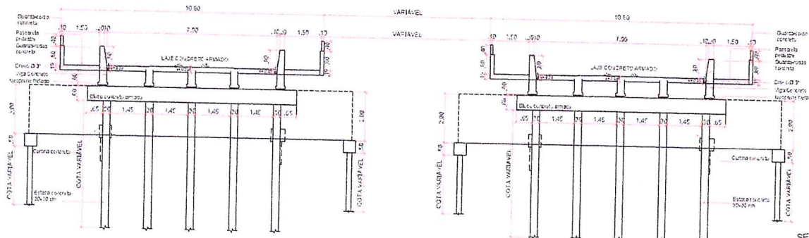
SEÇÃO 02 ESC. 1/100
