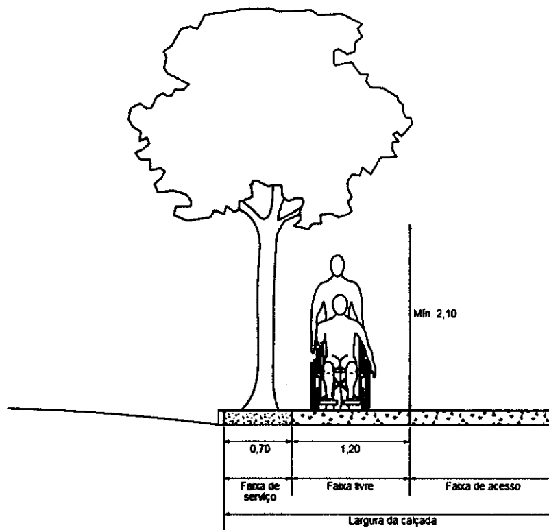
Figura 88 – Faixas de uso da calçada – Corte
