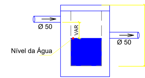
Corte Caixa de Gordura sem escala
