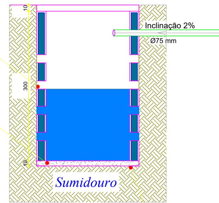
Detalhe Sumidouro sem escala
