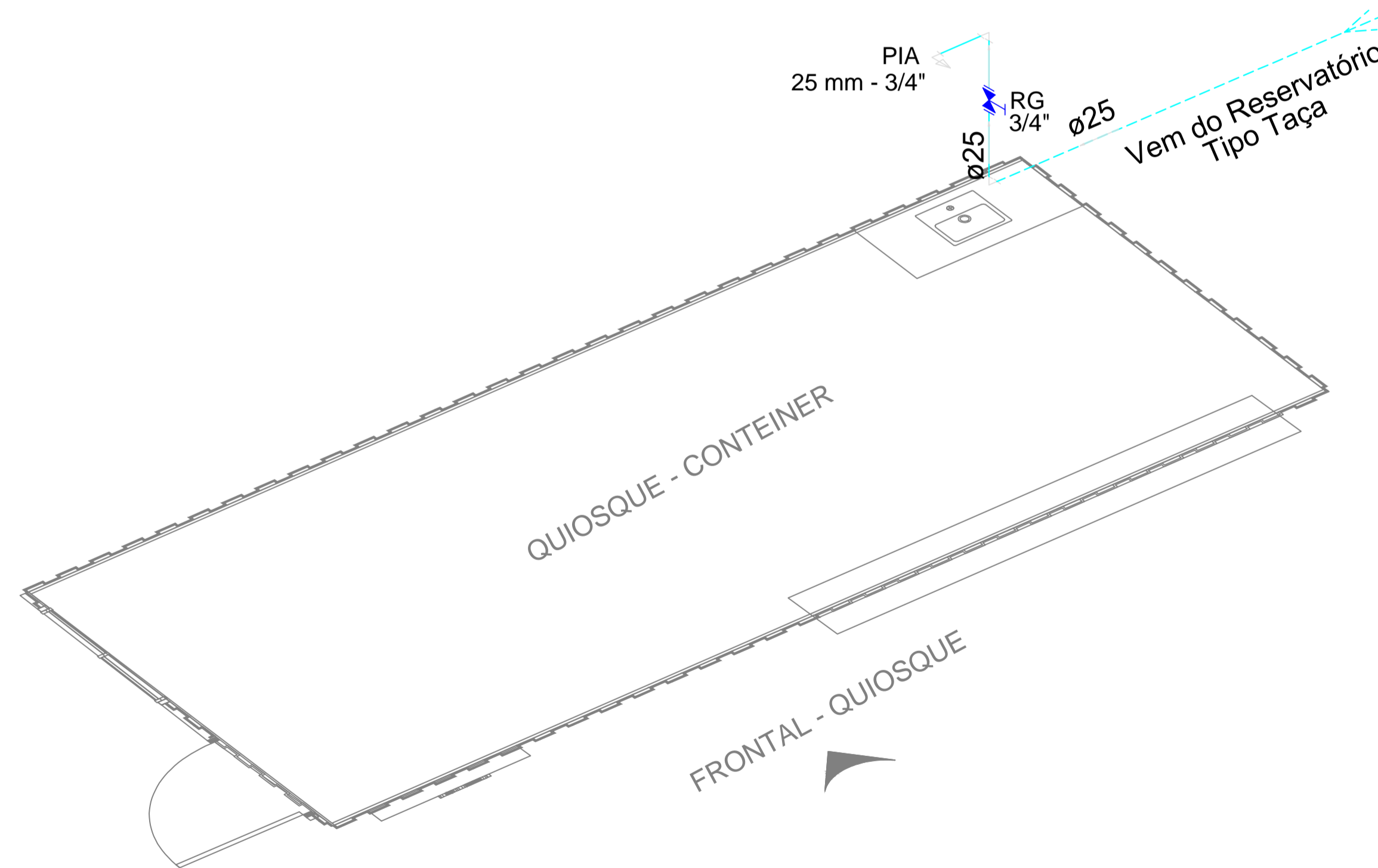
Detalhe hidráulico Isométrico QUIOSQUE escala 1:50
