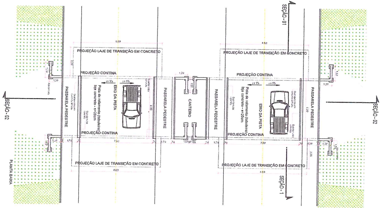
PLANTA BAIXA AV BRASIL ESC. 1/75
