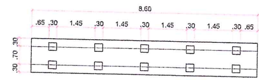
PLANTA - BLOCO CONCRETO ARMADO
