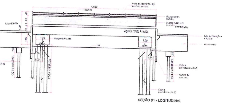
SEÇÃO 01 ESC. 1/75
