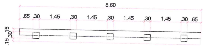
PLANTA - BLOCO CONCRETO ARMADO
