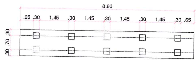
PLANTA - BLOCO CONCRETO ARMADO
