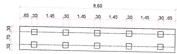
PLANTA BLOCO S/ESC.
