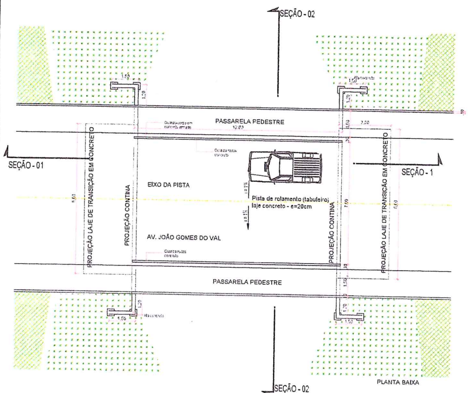
PLANTA BAIXA AV. PRES HUMBERTO C BRANCO ESC. 1/75
