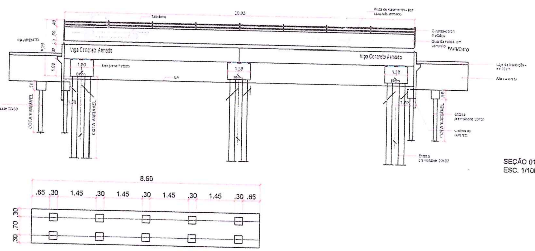
PLANTA - BLOCO CONCRETO ARMADO
