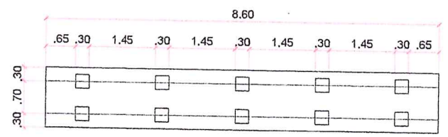
PLANTA - BLOCO CONCRETO ARMADO
