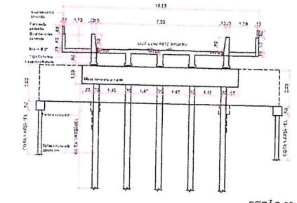
SEÇÃO 02 ESC. 1/100
