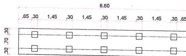
PLANTA - BLOCO CONCRETO ARMADO
