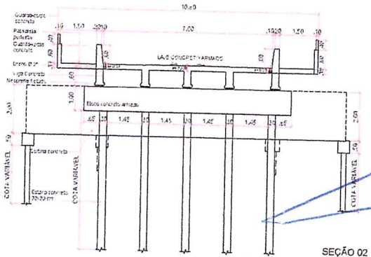
SEÇÃO 02 ESC. 1/75
