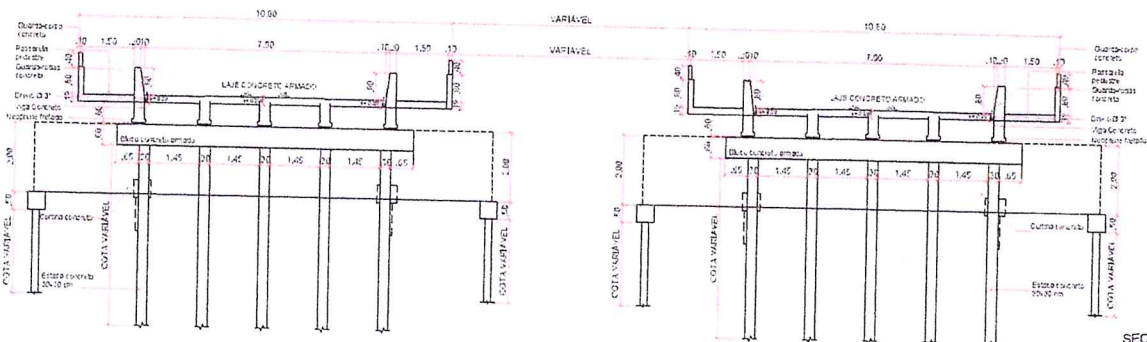
SEÇÃO 02 ESC. 1/100
