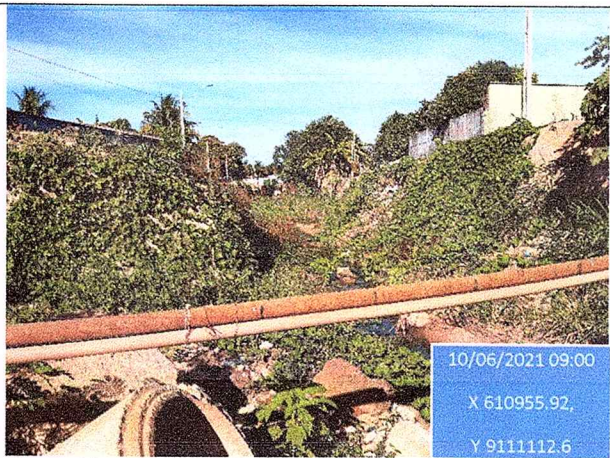
Figura 10 – Trecho da Etapa 02 do Canal Suprema Não Executada.
