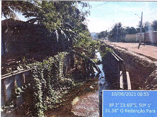
Figura 05 – Trecho da Etapa 02 do Canal Suprema Ferragem com Formas
