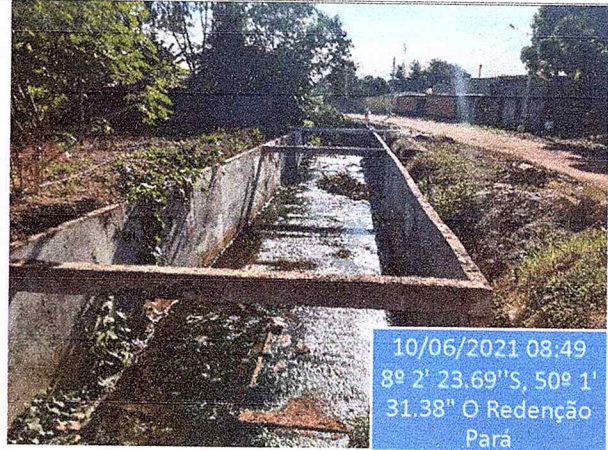
Figura 02 – Parte do Canal concretado da etapa 02 do Canal
